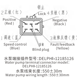
PWM 占空比调速模式 PWM Duty Cycle Speed Control Mode
