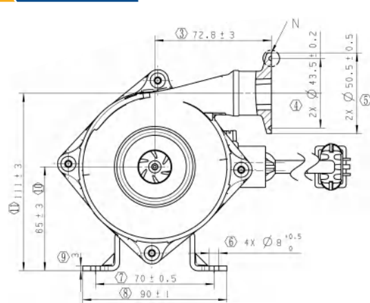
外形尺寸 Dimensions
