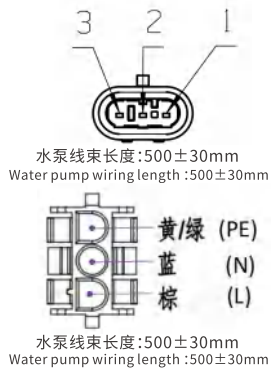
接插定义 Pinout
